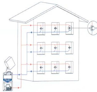
ESQUEMA DE CONEXIONES
